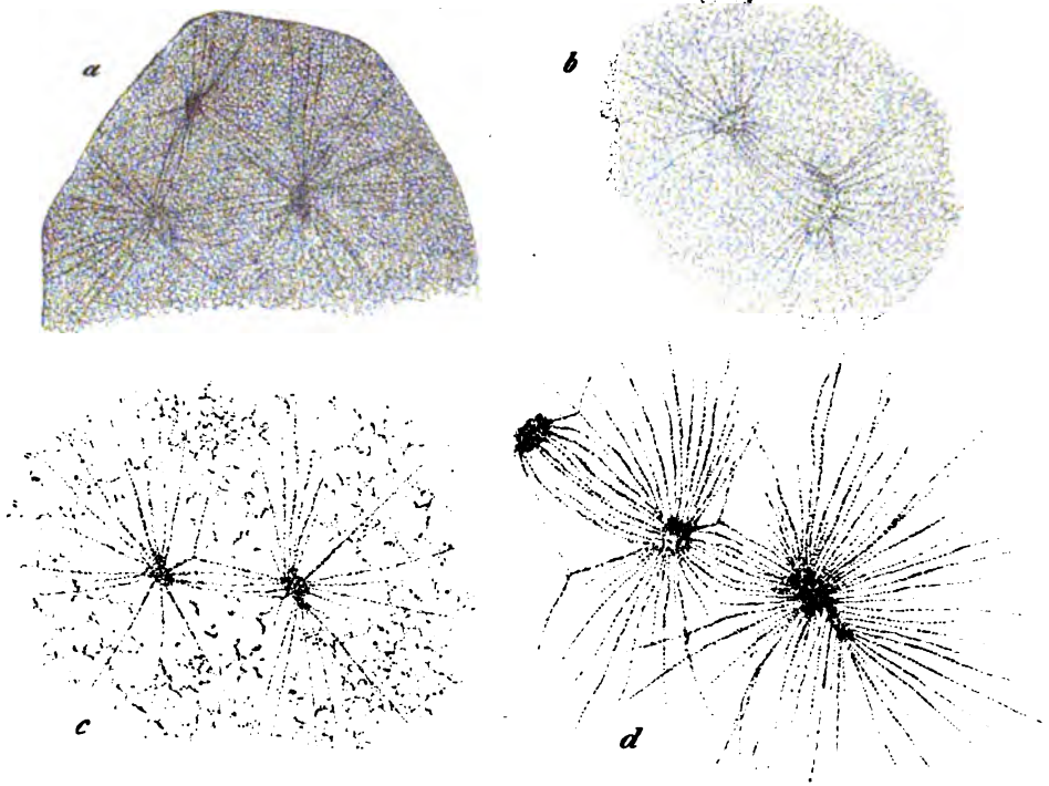
Fig. 13. Nachahmung karyokineticischer Figuren in Hollundermark. a 5-proc. Albumose in 5-proc. Gelatine; nach dem Erstarren der Gelatine wurden die Hollunderprismen in 1-proc. Osmiumsäure + 1-proc. Essigsäure eingelegt. Es waren drei kleine Inhaltsreste in der Markzelle, die als Ansatzpunkte für Strahlen aus Albumose gedient und das Ebenbild einer tripolaren Spindel hervorgeufen haben. Nachdem die Strahlen in der erstarrten Gelatine angeschossen waren, ist diese selbst engmaschig-gerüstig ausgefällt worden, ebenfalls von der Osmiumsäure. (Vergr. 600.) b 2-proc. Globulin, in schwachem Alkali (0,5 KOH) gelöst, mit Essigsäure gefällt und wieder gelöst und nun nach p. 207 in Hollundermarkschnitte injiziert; durch 0,75 KOH ausgefällt und mit 1-proc. Platinchlorid secundär fixiert. Die Strahlungen um die beiden Inhaltsreste und die sie einbettende gerüstige Fällung des Globulines waren von Kali erzeugt und sind ohne jede Veränderung von Platinchlorid conservirt worden (Vergr. 600). c 2-proc. Serumalbumin (in 0,2 KOH) in Hollunderschnitten mit FLEMMING'scher Lösung gefällt; die Strahlen sind hier homogener als es durch die Autotypie wiedergegeben ist; die lockere, aus schlängeligen Aggregaten winziger Globulite aufgebaute, an einigen Stellen dichter gehäufte Ausfällung würde bei dichterem Zusammenlagerung ein schönes protoplasmatisches Gerüstwerk gebildet haben. Man beachte auch die Verzweigungsstelle der Strahlen, rechts vom linken Ballen; zwei ebensolche Strahlen auch in der folgenden Figur (Vergr. 1000). d 2,5-proc. Albumose, leicht sauer, mit 1-proc. Osmiumsäure gefällt in einer Zelle, in der drei Kernreste hinter einander lagen. Dementsprechend sind auch die Strahlen angeordnet, die sich auch schön durchkreuzen; etwa 1 Sde. nach dem Einlegen eines imprägnirten Schnittes in Osmiumsäure auf den Objectträger. Die geringe Menge der Osmiumsäure hat nicht ausgereicht, um die zwischen den Strahlen noch vorhandene Albumoselösung ganz auszufällen, wesshalb die Strahlen, einige in der Figur weggelassene Körnchen abgerechnet, ganz frei liegen. (Vergr. 400.)
